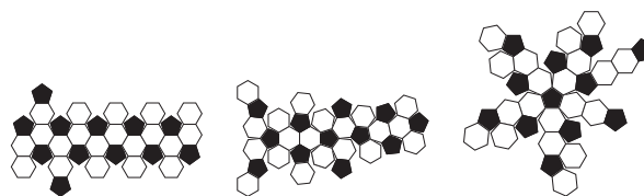
Figure 3. Trois patrons de l'icosaèdre tronqué.
